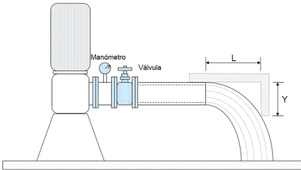
Figura 3.- Medición de flujo por el método de la escuadra.
